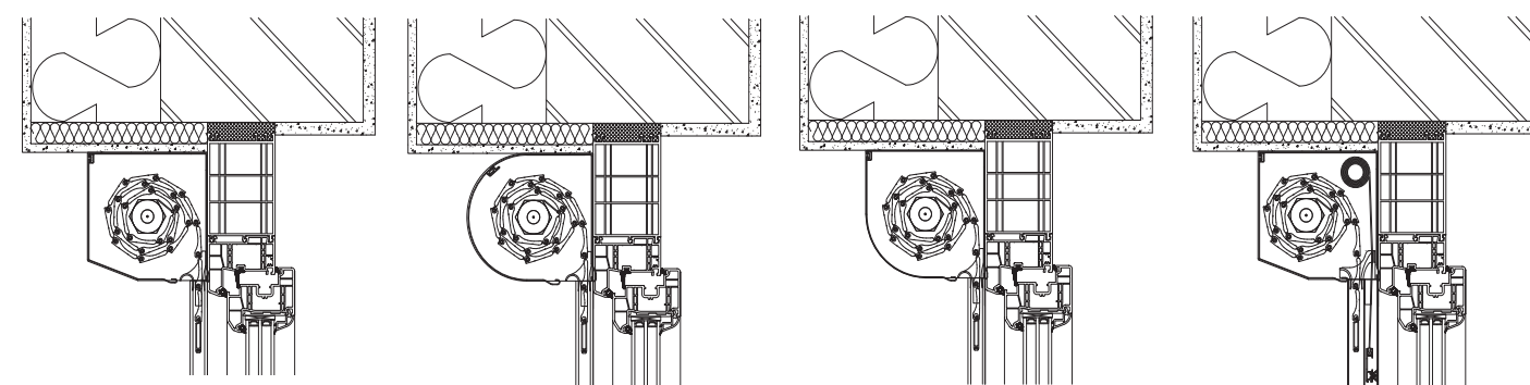
Obr. 1 - Roleta s boxem 20°
